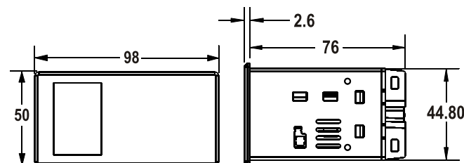
Panel Cutout : 92mm X 46mm (PID110-U)
